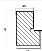
Rysunek techniczny
