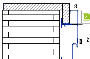
Ościeżnica Alu Hybrid
