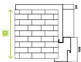
Rysunek techniczny
