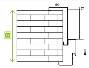
Rysunek techniczny
